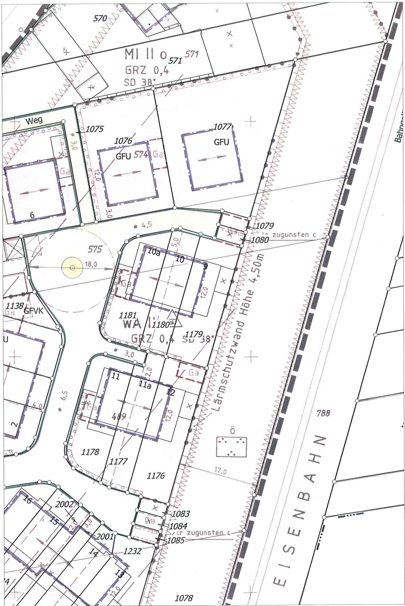
Bebauungsplan ausschnitt S 137 1:500
